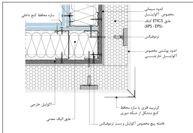
ETICS1: اتصال کتف خارجی با ساختار ETICS
