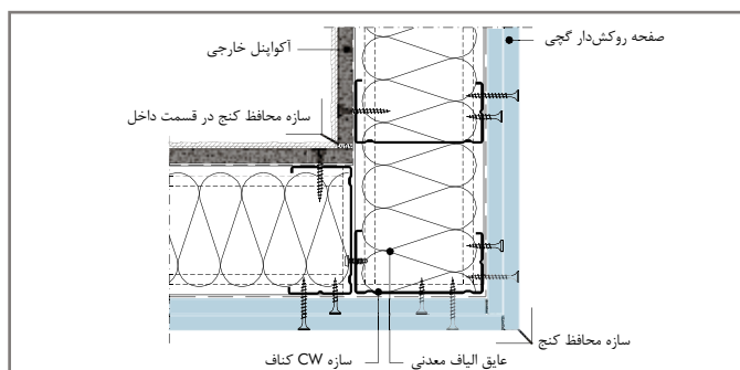
W384E-D1 اتصال کج داخلی
