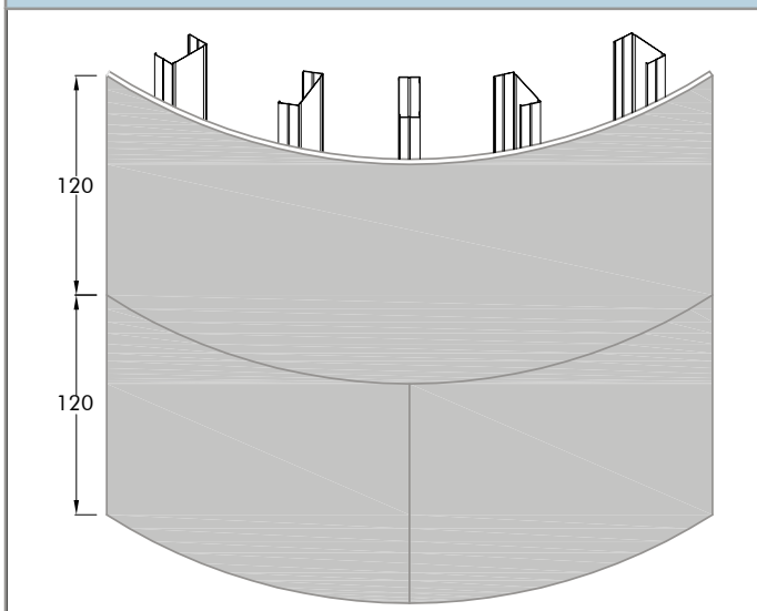
اجرا با پنل به عرض ۱۲۰cm تا حداکثر شعاع قوس ۳m
