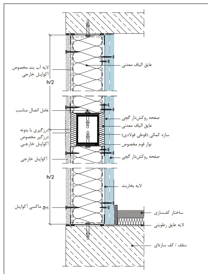
مقطع عمودی دیوار خارجی آکوپنل با استفاده از قوطی‌کشی فلزی در وسط ساختار
