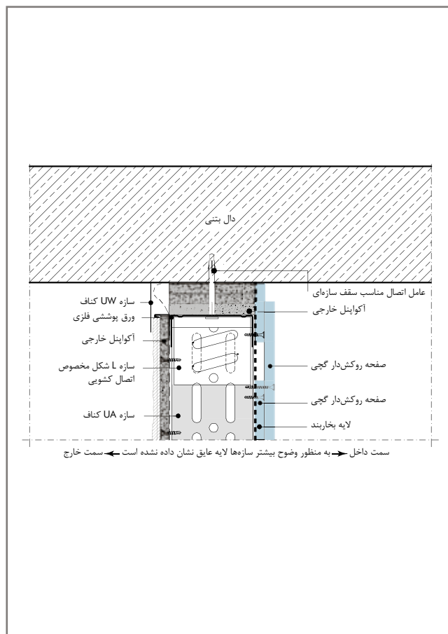
گزینه ۱: W384E-VOG1 اتصال کشویی لغزان به سقف سازه‌ای
