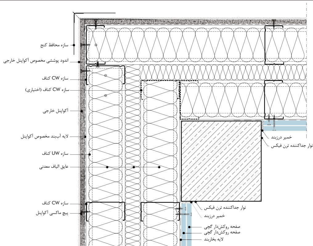
W388E-ES1 اتصال کنج خارجی سطح مقطع افقی
