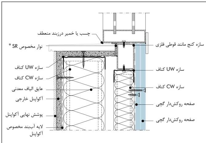
W388E-FE - VU1 گزینه ۱: اتصال دیوار خارجی آکوابنل به قاب پایین پنجره
