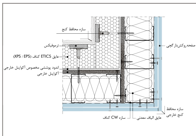
ETICS1: دیوار خارجی به همراه عایق الیاف معدنی و ETICS
