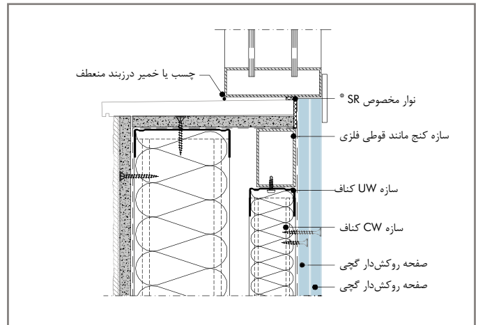
W388E-FE - VU2 گزینه ۲: اتصال دیوار خارجی آکوابنل به قاب پایین پنجره
