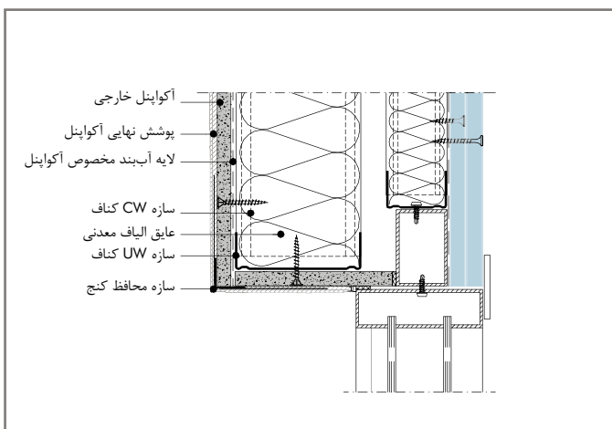
W388E-FE - VO1 گزینه ۱: اتصال دیوار خارجی آکوابنل به قاب بالای پنجره
