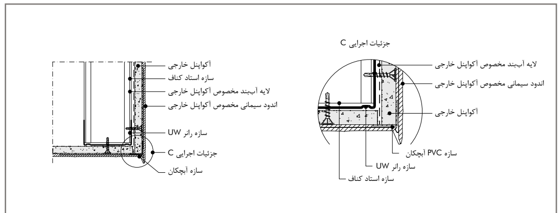
سازه مخصوص انتهایی اندودکاری (آبچکان) از جنس PVC
