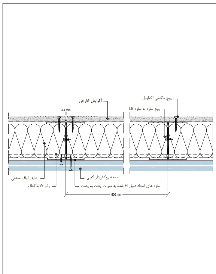
پلان دیوار خارجی آکوپنل با استفاده از سازه استاندارد CW دبل H
