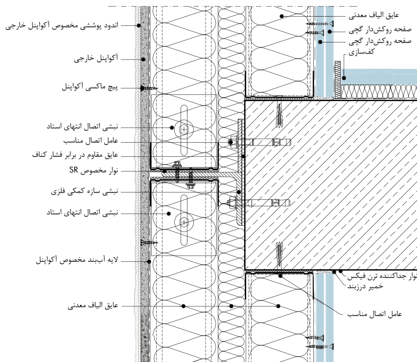
W388E-VM2 گزینه ۲: اتصال به سقف در تراز طبقات با استفاده از ورق و نبشی فولادی
