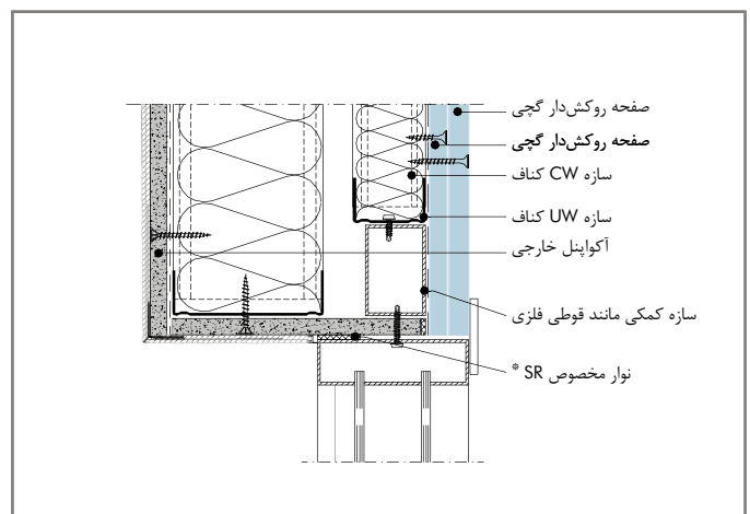
W388E-FE - VO2 گزینه ۲: اتصال دیوار خارجی آکوابنل به قاب بالای پنجره
