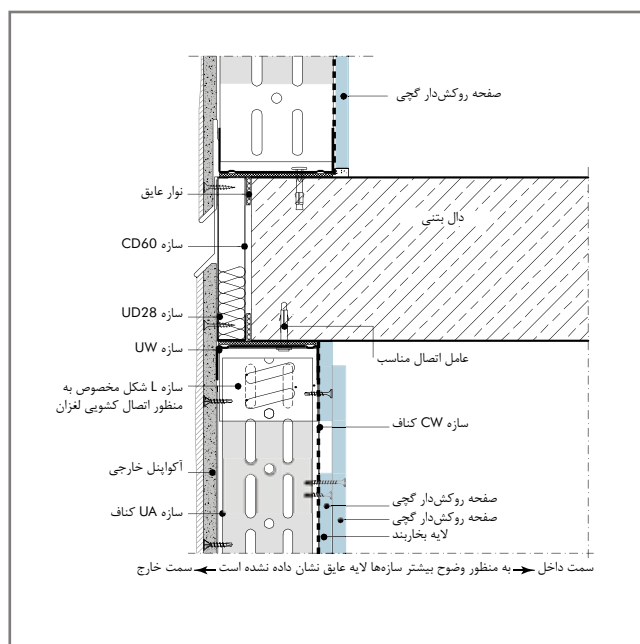
گزینه ۱: W384E-VMG1 اتصال کشویی لغزان به سقف سازه‌ای
